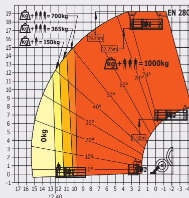
Погрузчик с выставленными стабилизаторами с платформой (модель MT-X 1840 A)
