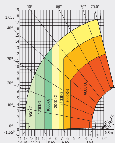
Погрузчик с выставленными стабилизаторами с вилами
